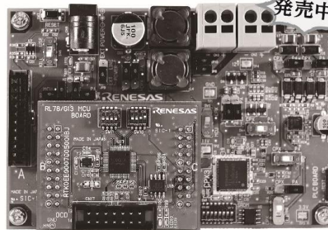
低電圧版 (DC16V-48V) PLC 評価ボード RTK0EE0007D02001BJ
