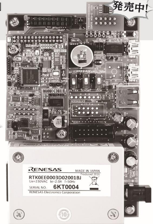
高電圧版 (AC100V-230V) PLC 評価ボード RTK0EE0003D02002BJ
