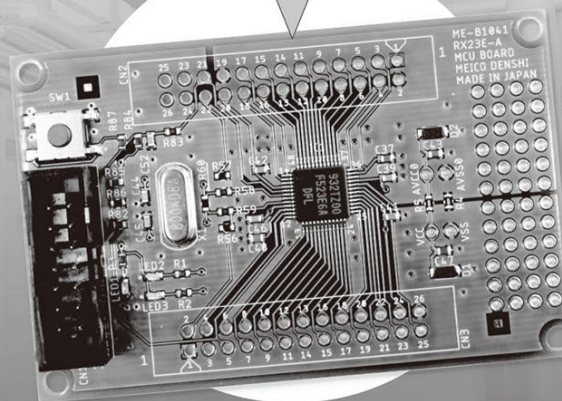
RX23E-A (型式:ME-B1041)
